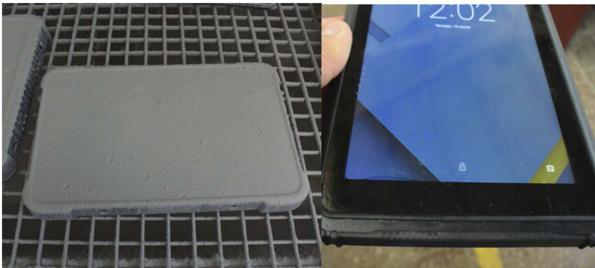
Фото 1. Проведение испытаний.
